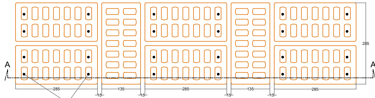
PRIMO CORSO DI MATTONI IN PIANTA (ZONA RETTILINEA)
