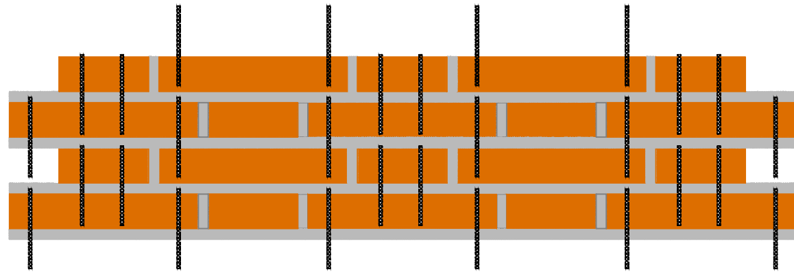
PRIMO CORSO DI MATTONI IN PIANTA (ZONA RETTILINEA)
