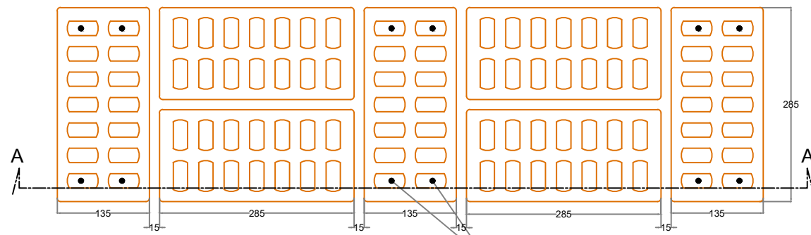
SECONDO CORSO DI MATTONI IN PIANTA (ZONA RETTILINEA)
