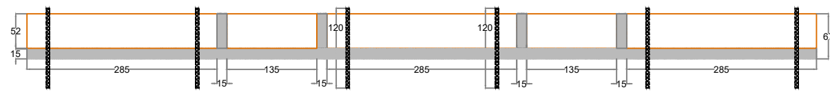
SEZIONE A-A
