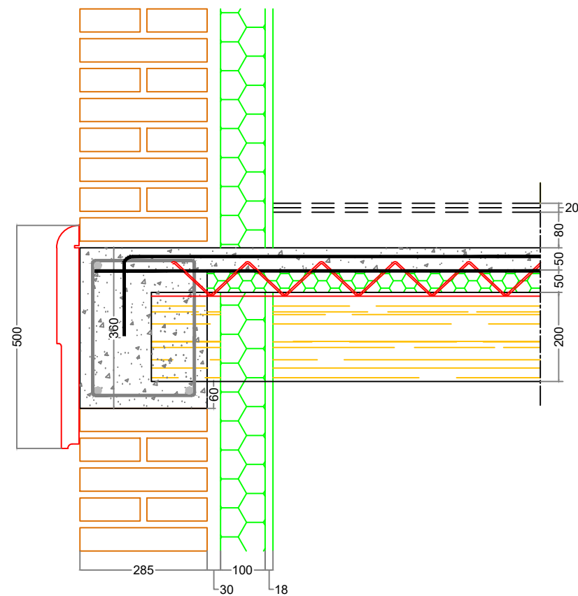
SOLAIO COMPOUND TRAVETTO S3 10x20
