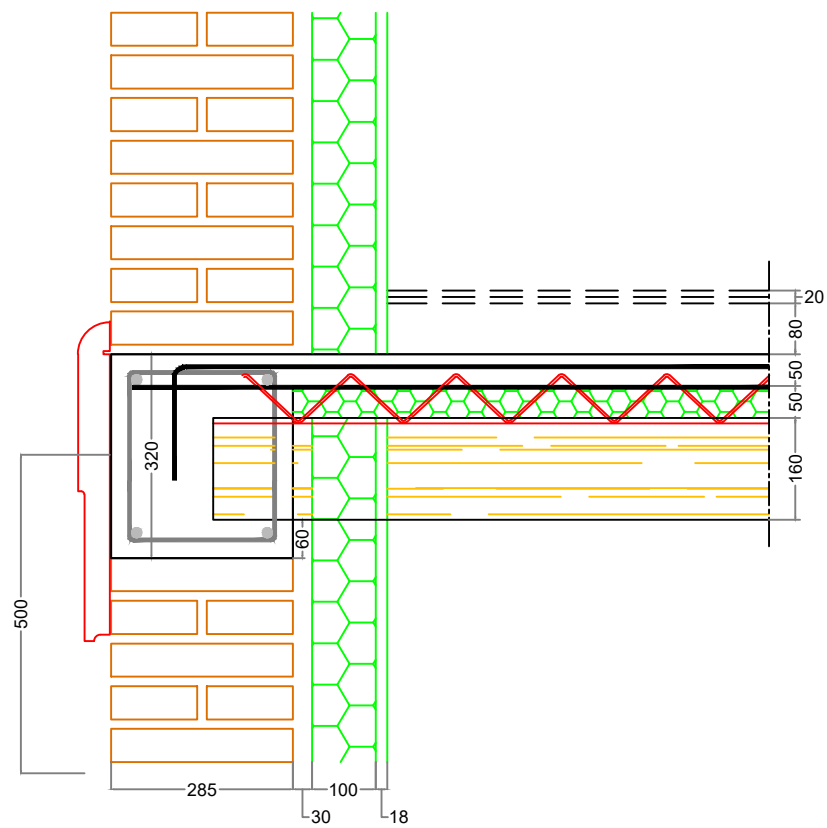
SOLAIO COMPOUND TRAVETTO S2 10x16
