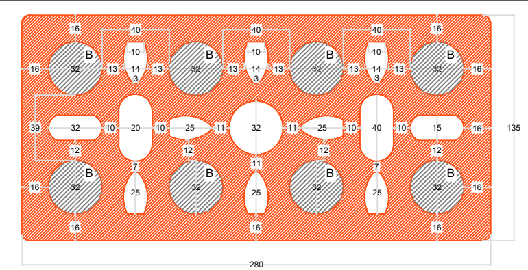
Terzetto Bolognese: 280x135x75 (Percentuale di foratura 32%)
