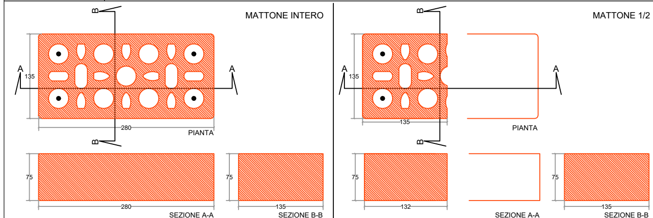
Terzetto Bolognese: 280x135x75 (Percentuale di foratura 32%)
