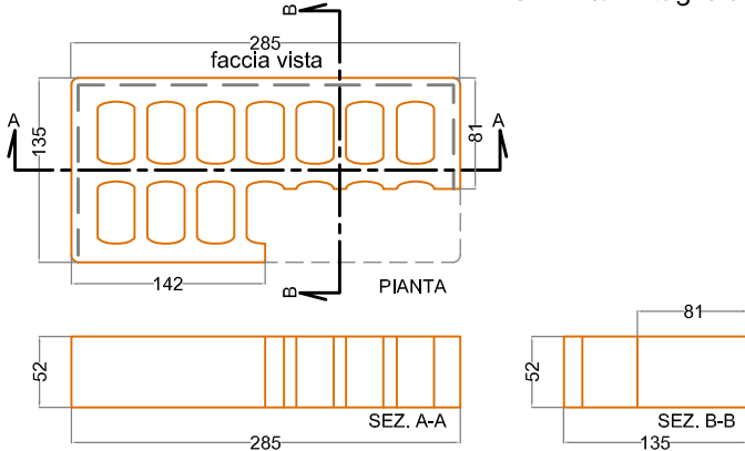
MATTONE 3/4 - taglio a L
