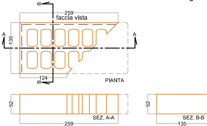
MATTONE 3/4 - taglio 45°
